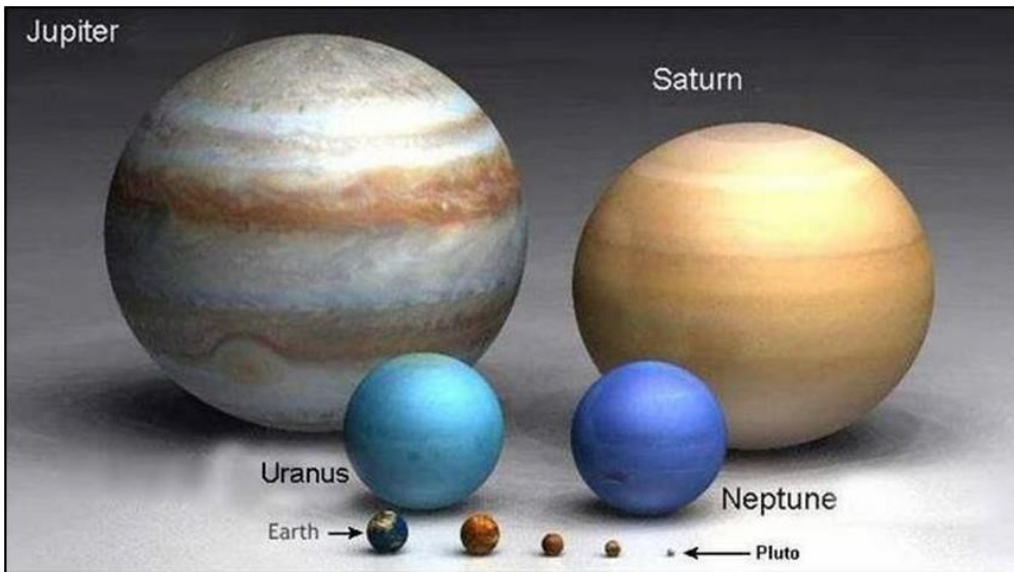
Planete se groottes t.o.v. mekaar
