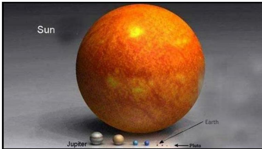
Planete se groottes t.o.v. Ons Son
